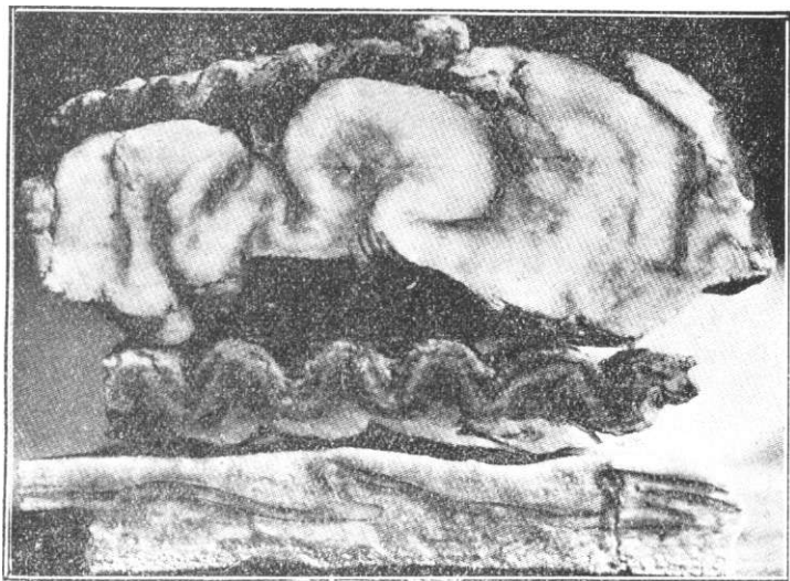
2. kép. Gyűrött gipsz rétegek. Az alsónál érdekes, hogy a gyűrött réteghez két szomszédos rétege plasztikusan idomul. A második szép szabályos redőkhöz gyűrű durva szemcsés gipsz réteg, alsó szomszédja rostos gipsz, mely a ráncosító erő hatására lépcsőzetesen elvetődött. A harmadik alabástromszerű gipsz, begyűrű márga anyagokkal. Jobb és bal végén a gyűrődés meglehetősen elmosódott. A legfelső gyűrődött réteg csak 3 mm. vastagságú. \frac{1}{2} term. nagyság.
