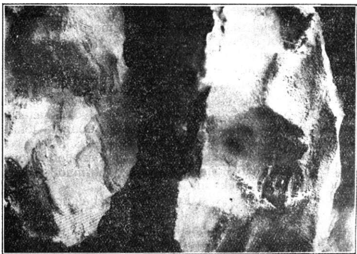
1. kép. Kettéfürészelt tisztátalan tömör gipszdarab. Baloldali felén kivehetők a repedések és egy fehér alabástrommal kitöltött kockalakú üreg. A jobb oldali felén a deformált kocka alakú üregből majdnem egészen ki van oldva az alabástrom. 1/3 term. nagyság.
